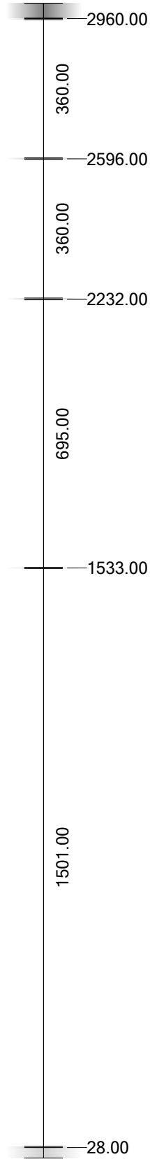
30/34 -- Volige, 23.00 x 180.00 mm -- 3000.00 mm -- Exemple unique
