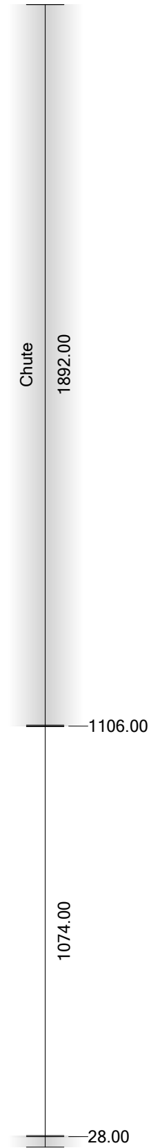
25/34 -- Poteau, 160.00 x 160.00 x 3000.00 mm -- Exemple unique
