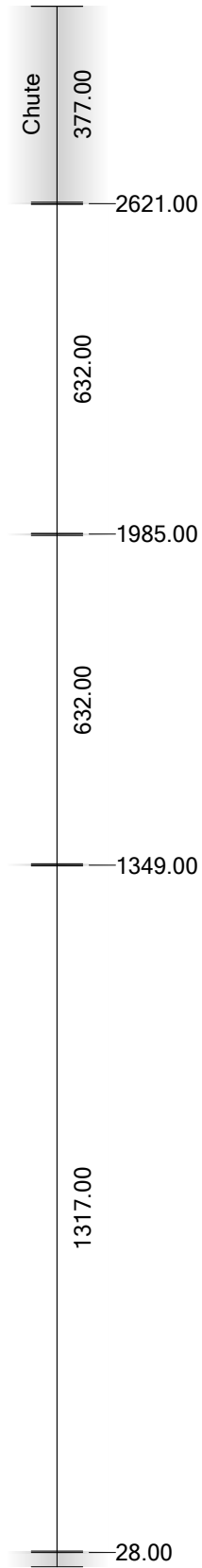
24/34 -- Poteau, 160.00 x 160.00 x 3000.00 mm -- Exemple unique
