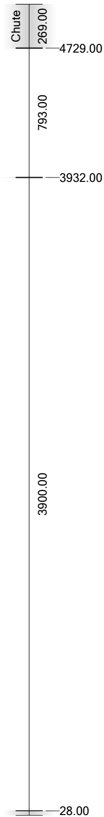
1/34 -- Bandeau, 40.00 x 180.00 -- 5000.00 mm -- Exemple unique
