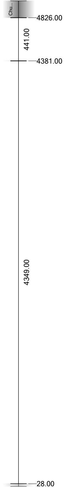
9/34 -- Chevron/Entretoise, 55.00 x 160.00 -- 5000.00 mm -- Exemple unique
