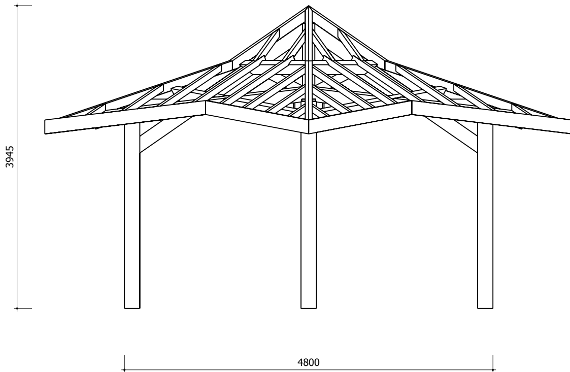
COUPE A-A
