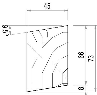
Vue par bout du chevron biai
