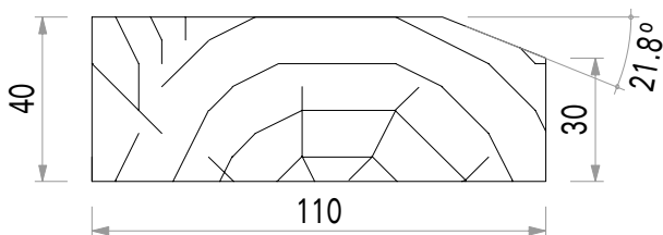
Vue par bout du faitage
