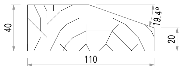
Vue par bout de la sablière
