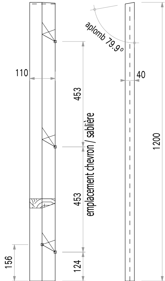
Vue par bout de la sablière
