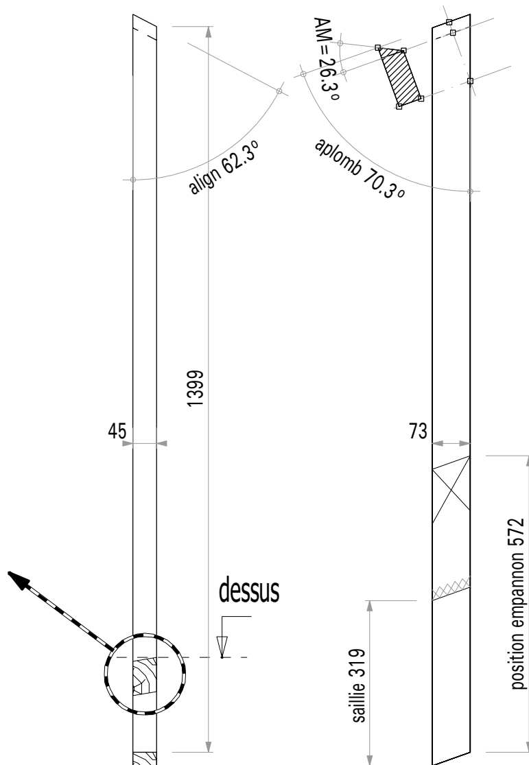
Vue par bout du chevron biai
