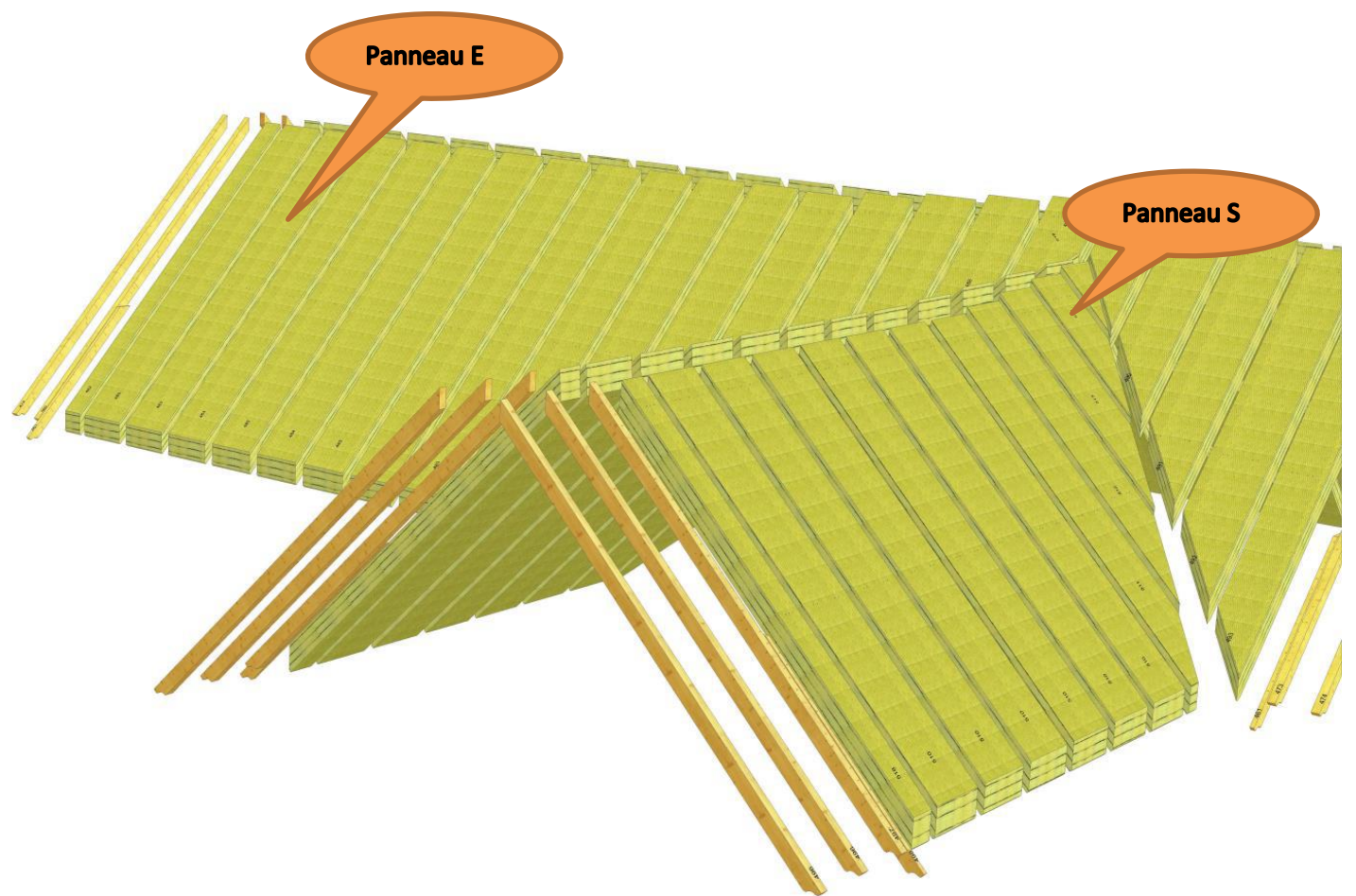
Perspective éclatée des panneaux de toiture et des chevrons de rives.
