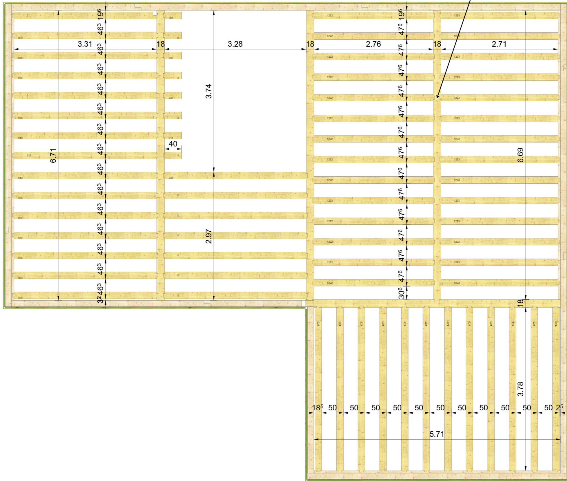
VUE EN PLAN SOLIVAGE
