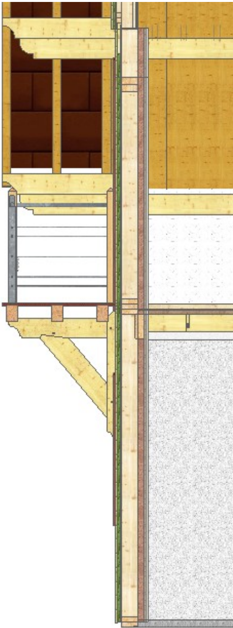
Coupe verticale d'un mur d'ossature
