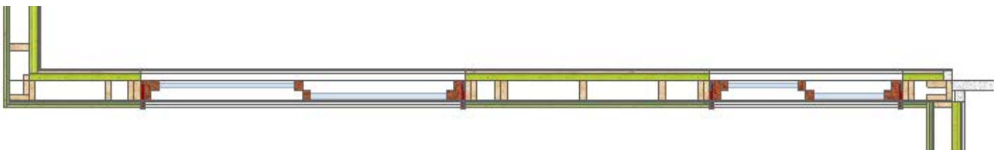
Coupe horizontale d'un mur d'ossature
