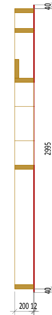
Coupe A-A
