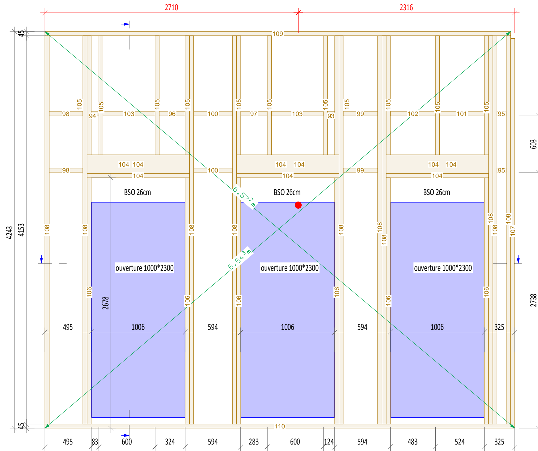
Coupe A-A
