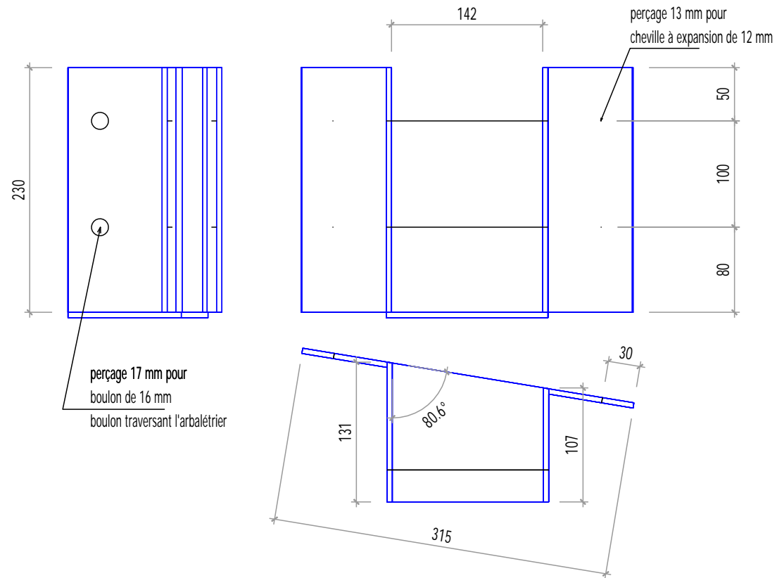
Ferrure F7 Boitier mécano soudé - Ferme 5
