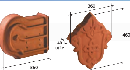
About de rive universelle droite à emboîtement Réf. 1073
