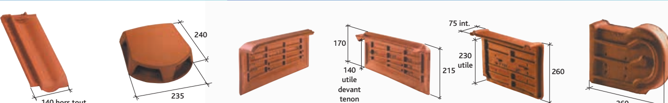
1/2 tuile Provinciale Réf. 212.01
