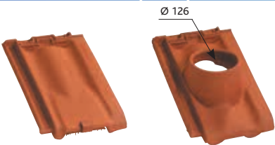
Tuile de ventilation Provinciale (section avec grille = 13 cm²) Réf. 212.20
